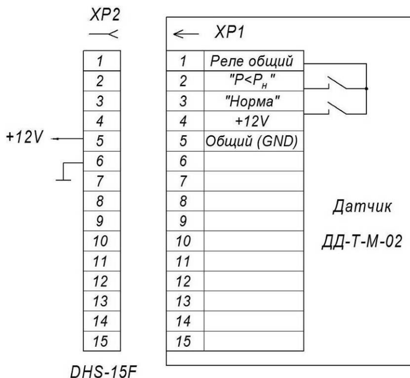
Рисунок 1.26 – Электрическая схема подключения датчика давления DD-T-M-02
