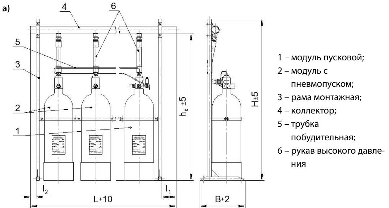
Рисунок 2.1 – Схема однорядной батареи из модулей МГП (60-A-d), МГП (65-A-d) «АТАКА» или «АТАКА 3»:
