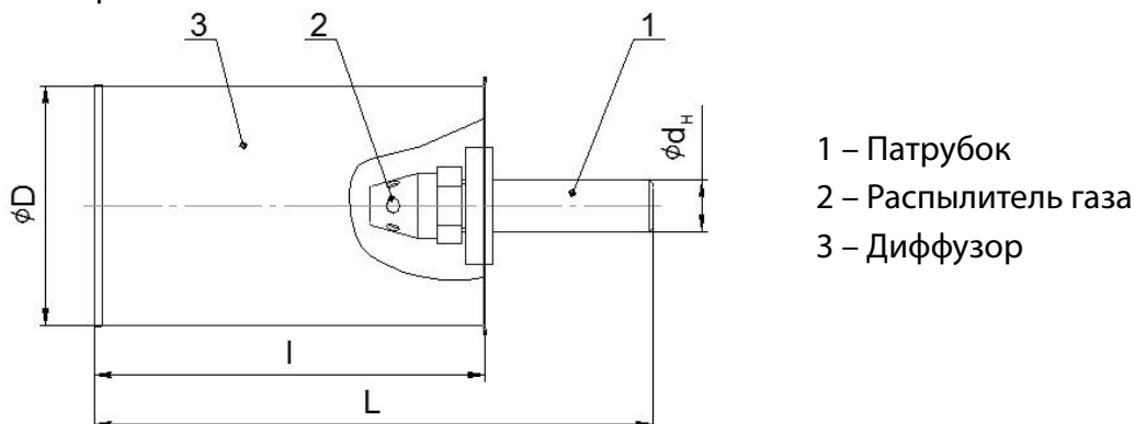
Рисунок 4.2 – Устройство РЛП
