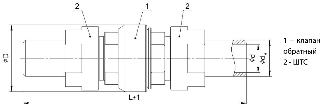
Рисунок 6.1 – Клапан обратный с ШТС
