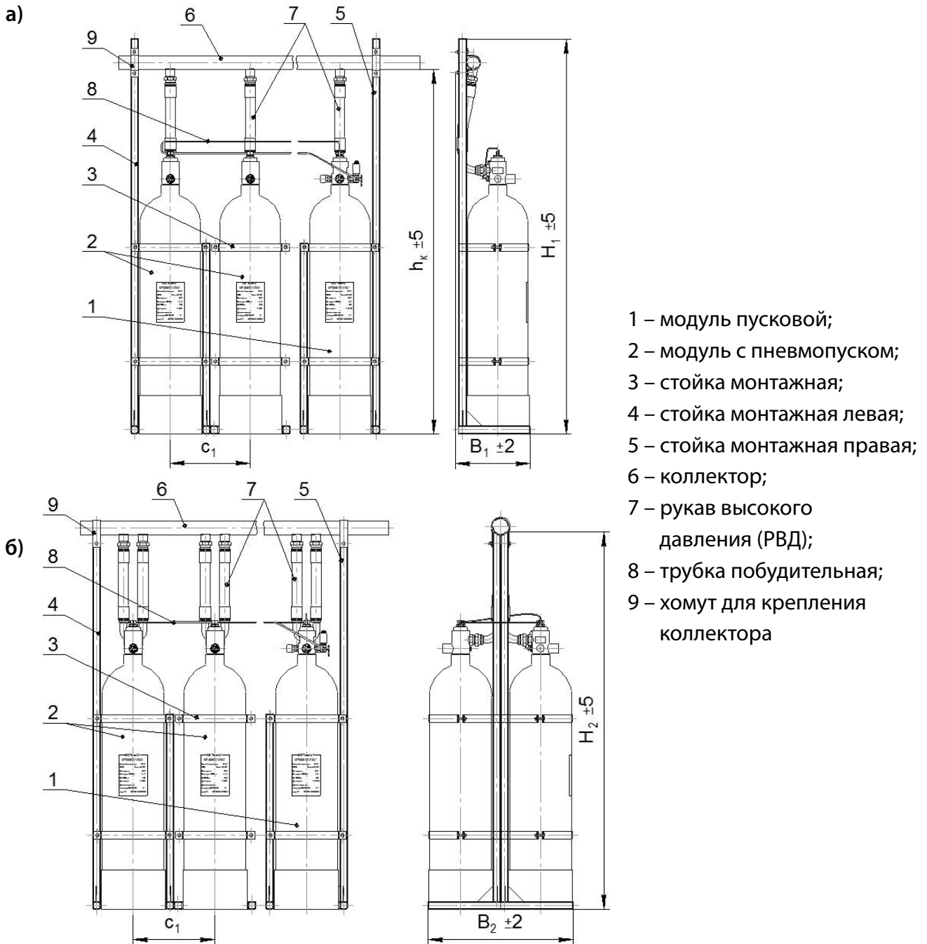
Рисунок 2.8 – Схема батареи на стойках монтажных из модулей МГП (60-А-d) или МГП (65-А-d) «АТАКА» или «АТАКА 3»: а) однорядная; б) двухрядная
