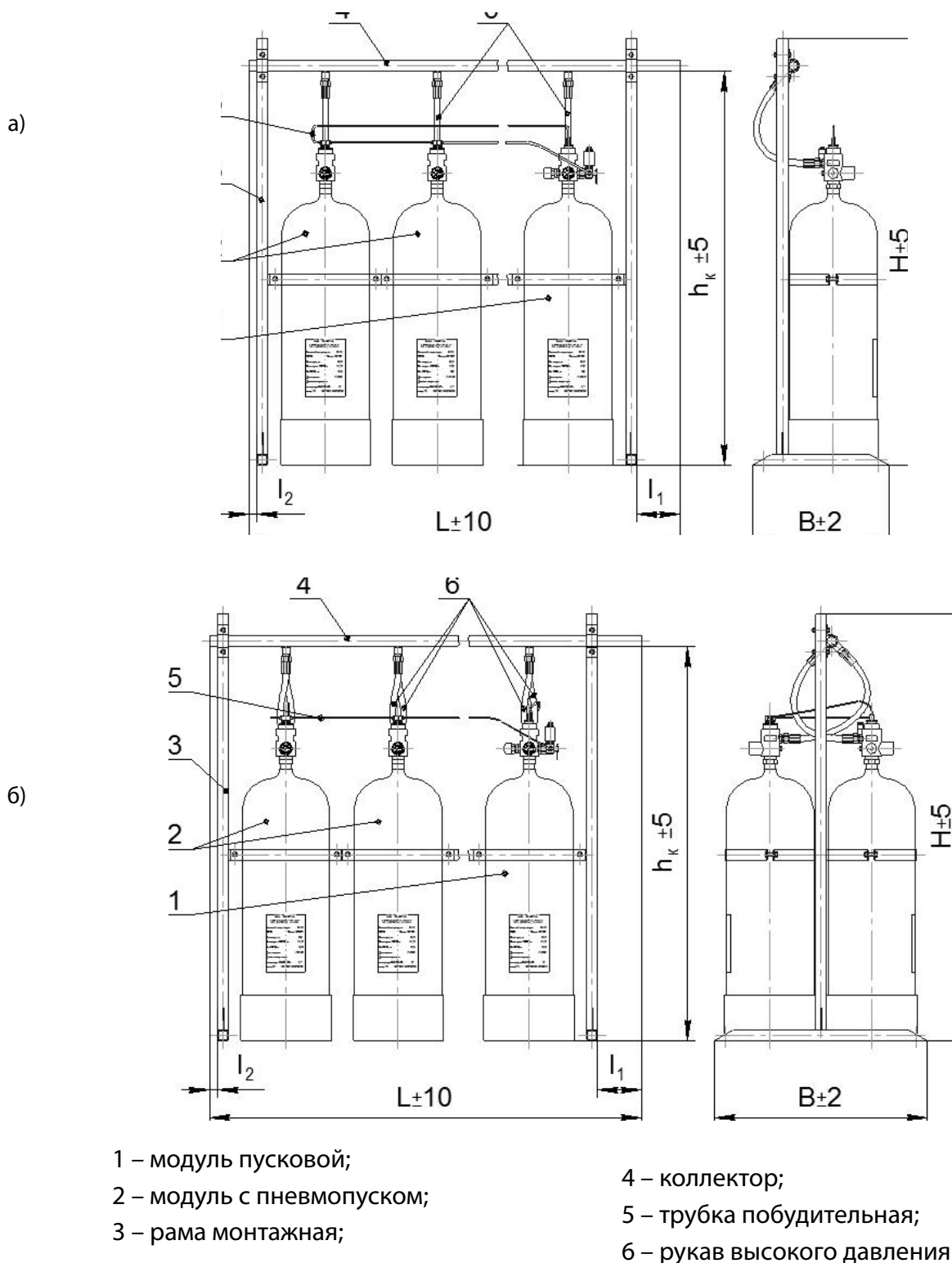
Рисунок 2.3 – Схема батареи из модулей МГП (150-А-15), МГПи (150-А-15) «АТАКА» или МГП (150-А-15) «АТАКА 3» или МГП (150-А-15) «АТАКА 2»: а) однорядная батарея; б) двухрядная батарея
