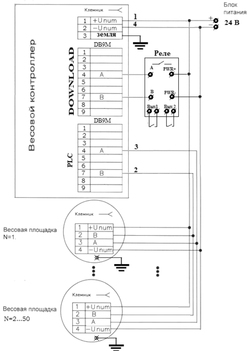
Рисунок 1.21 – Схема подключения УКМ-2
