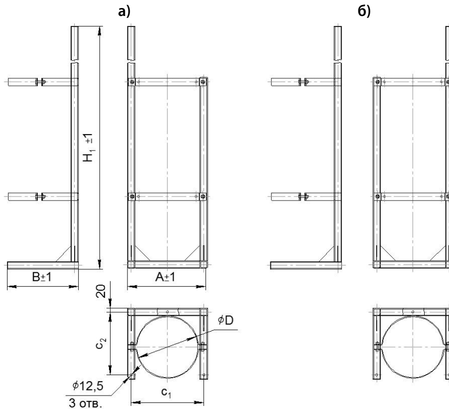
Рисунок 3.5 – Стойка монтажная в составе однорядной батареи «АТАКА» или «АТАКА 3»: а) левая, б) правая
