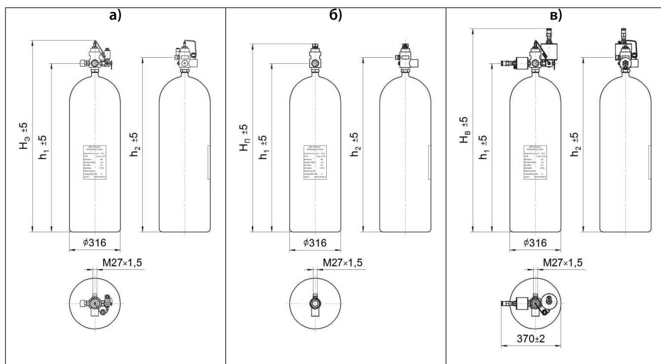
Рисунок 1.16 – МГПи (150-А-15), основанные на стальных бесшовных баллонах: а) с электрическим и ручным пуском; б) с пневмопуском; в) взрывозащищенный
