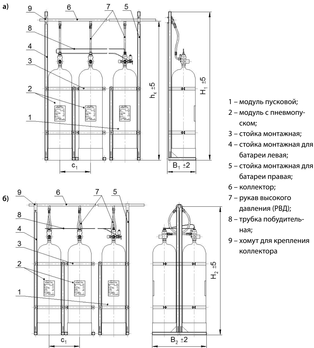
Рисунок 2.9 – Схема батареи на стойках монтажных из модулей МГП (150-А-15), МГПи (150-А-15) «АТАКА», МГП (150-А-15) «АТАКА 2» и МГП (150-А-15) «АТАКА 3»:
