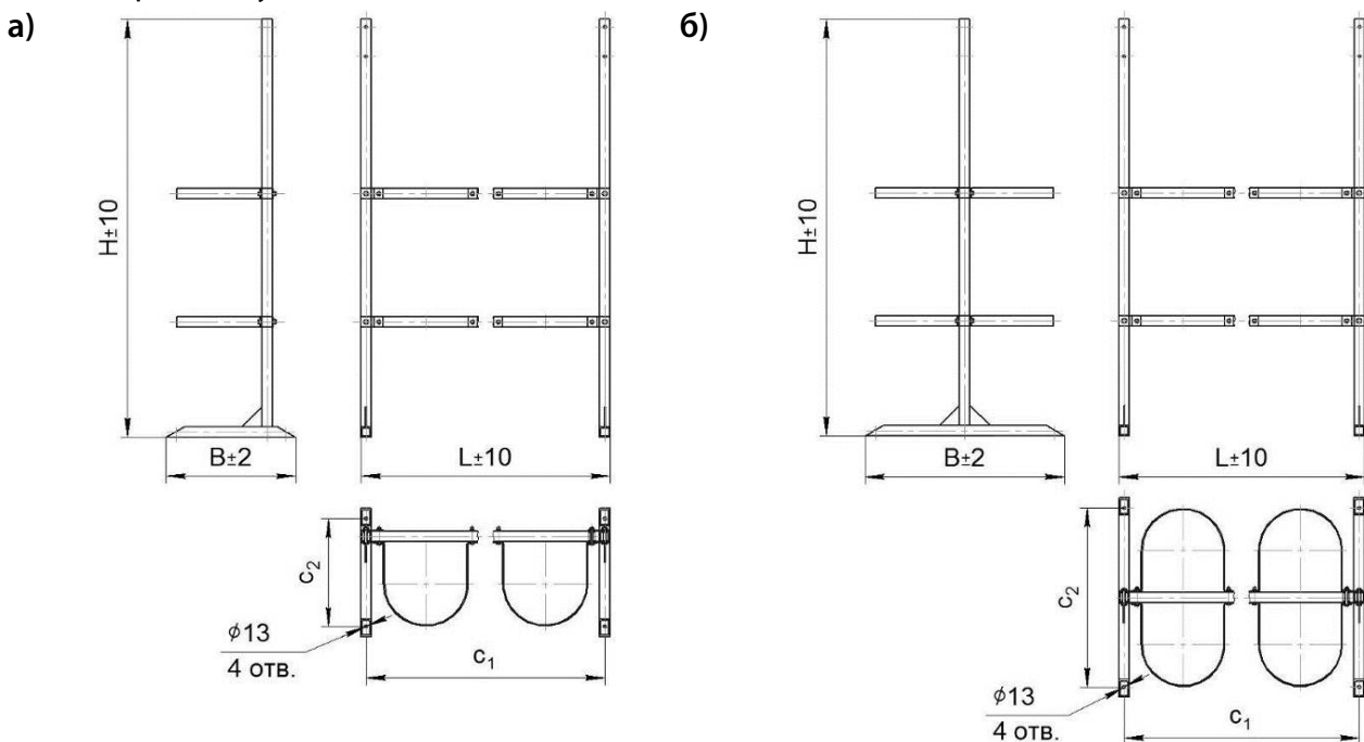
Рисунок 3.9 – Рама монтажная:
