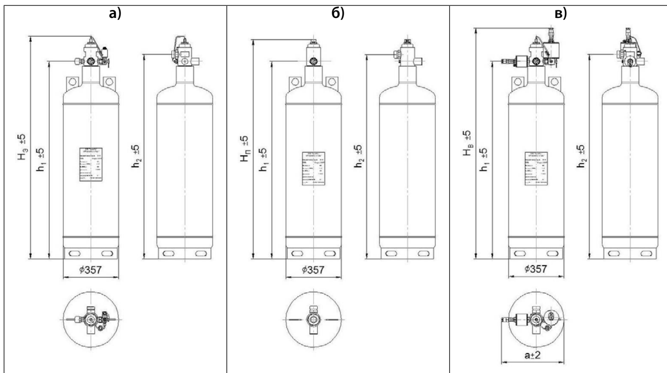
Рисунок 1.8 – МГП (65-A-d), основанные на стальных штампованных баллонах: а) с электрическим и ручным пуском; б) с пневмопуском; в) взрывозащищенный
