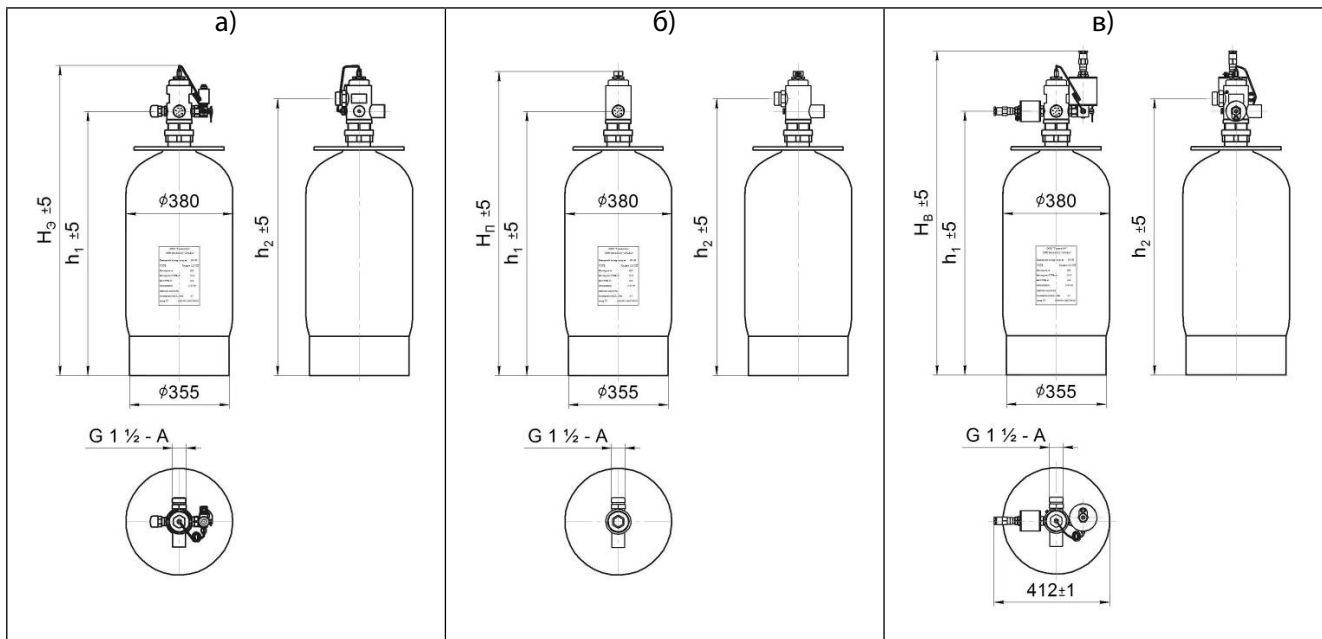
Рисунок 1.6 – МГП (60-А-d), основанные на металлокомпозитных баллонах: а) с электрическим и ручным пуском; б) с пневмопуском; в) взрывозащищенный
