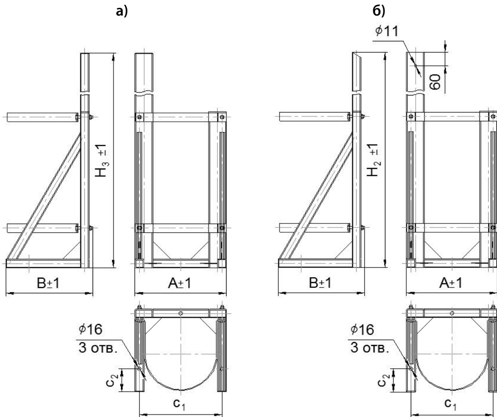
Рисунок 3.8 – Стойка монтажная усиленная:
