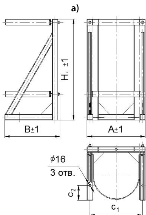
Рисунок 3.7 – Стойка сейсмостойкая монтажная для отдельно стоящих модулей и промежуточных модулей в составе батареи
