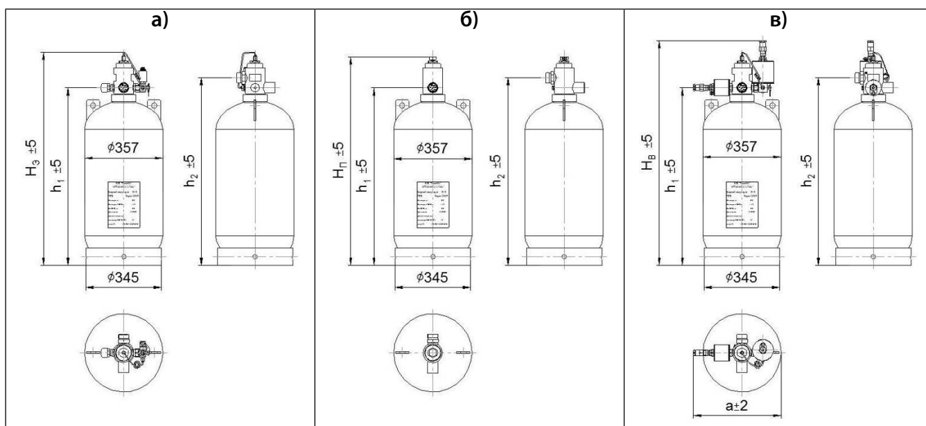
Рисунок 1.9 – МГП (65-A-d), основанные на стальных сварных баллонах: а) с электрическим и ручным пуском; б) с пневмопуском; в) взрывозащищенный
