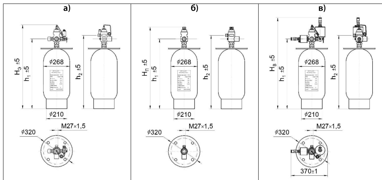
Рисунок 1.13 – МГП (150-20-15), основанные на композитных баллонах:
