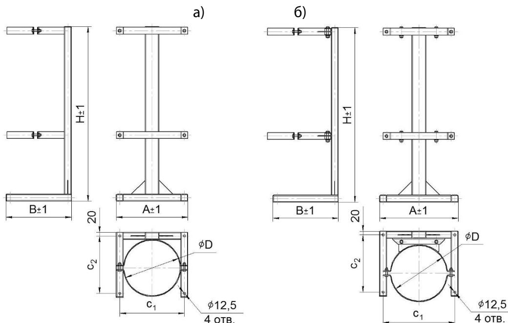
Рисунок 3.4 – Стойка монтажная:
