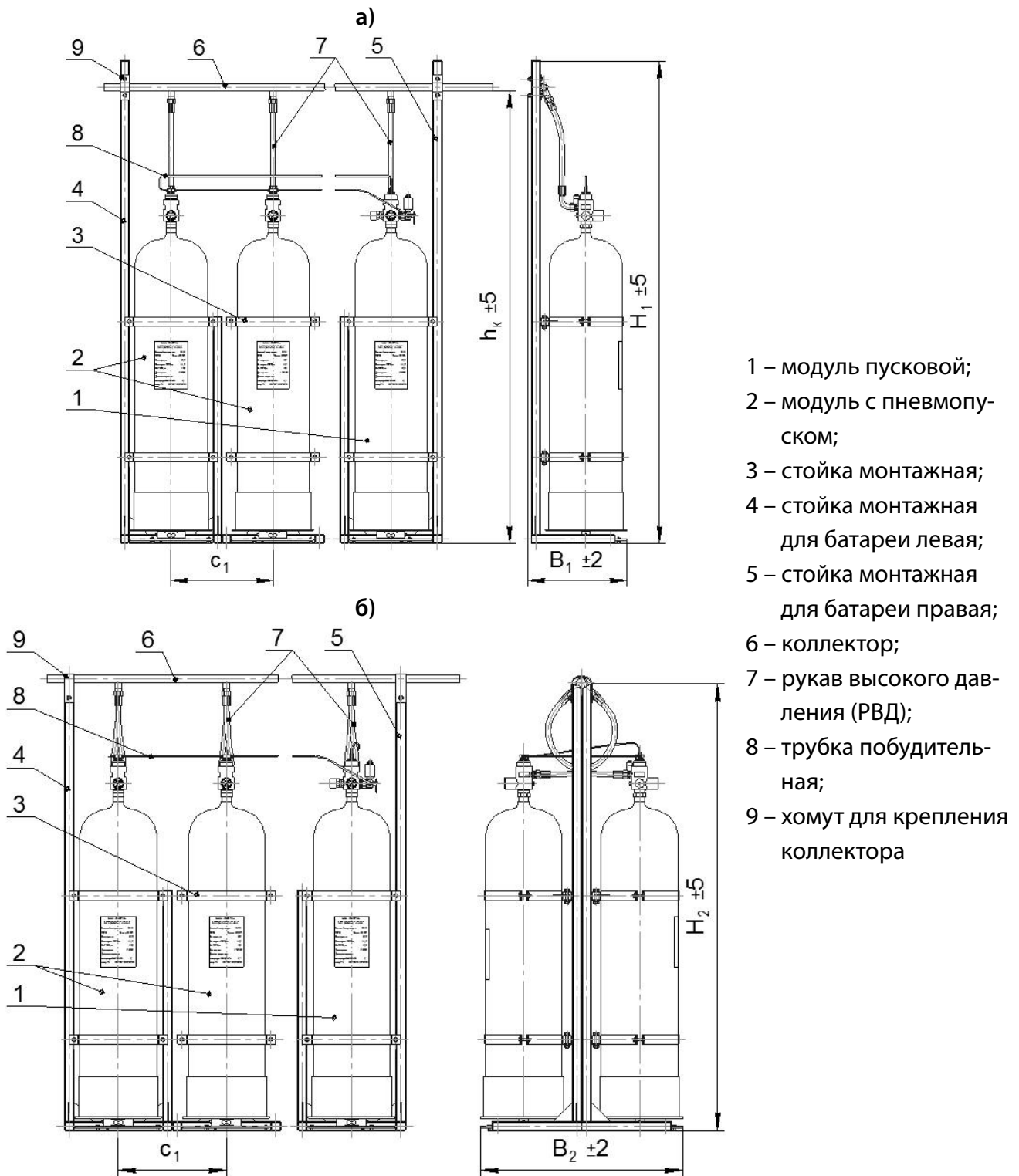
Рисунок 2.10 – Схема батареи на стойках монтажных из модулей МГП (150-А-15) «АТАКА 1»: а) однорядная; б) двухрядная
