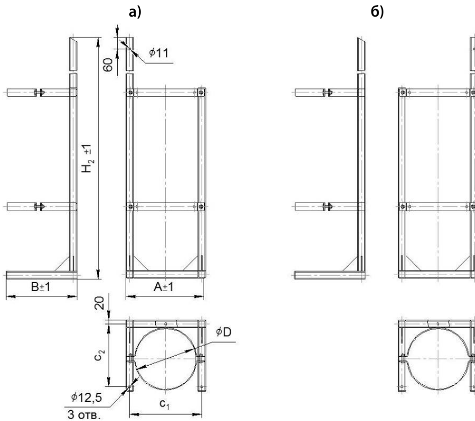
Рисунок 3.6 – Стойка монтажная в составе двухрядной батареи «АТАКА» или «АТАКА 3»: а) левая, б) правая
