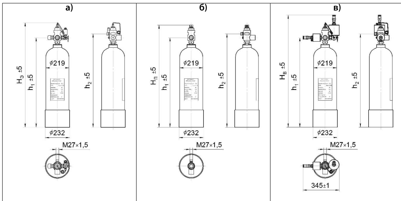
Рисунок 1.12 – МГП (150-20(25, 40)-15), основанные на стальных цельнотянутых баллонах: а) с электрическим и ручным пуском; б) с пневмопуском; в) взрывозащищенный
