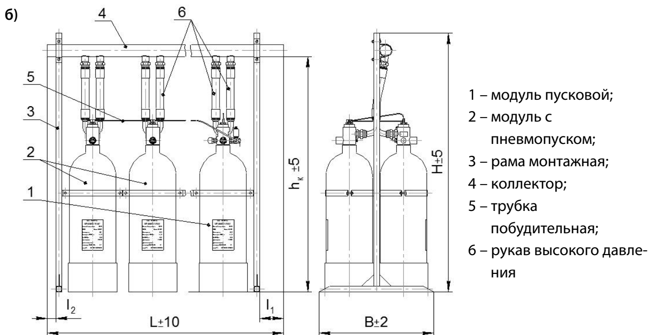
Рисунок 2.2 – Схема двухрядной батареи из модулей МГП (60-А-d), МГП (65-А-d) «АТАКА» или «АТАКА 3»
