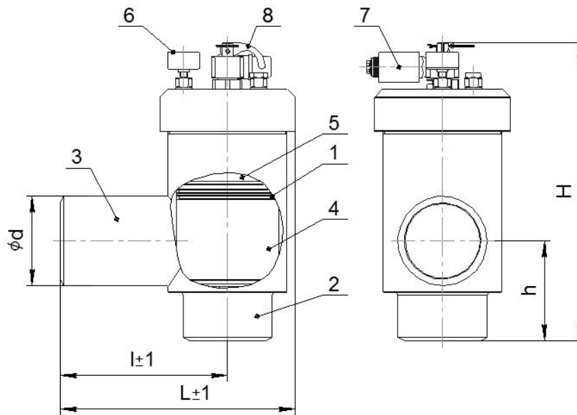
Рисунок 6.3 – Устройство распределительное исполнения 2
