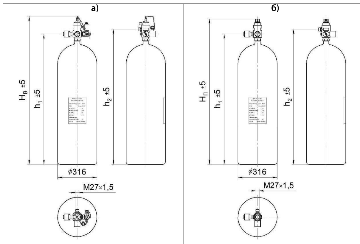
Рисунок 1.31 – МГП (150-А-15), основанные на стальных бесшовных баллонах: а) с электрическим и ручным пуском; б) с пневмопуском
