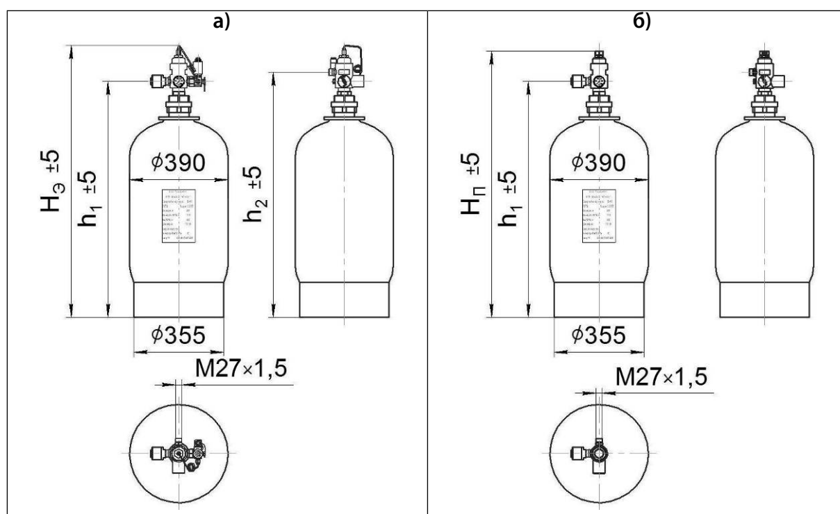
Рисунок 1.30 – МГП (150-А-15), основанные на металлокомпозитных баллонах: а) с электрическим и ручным пуском; б) с пневмопуском.
