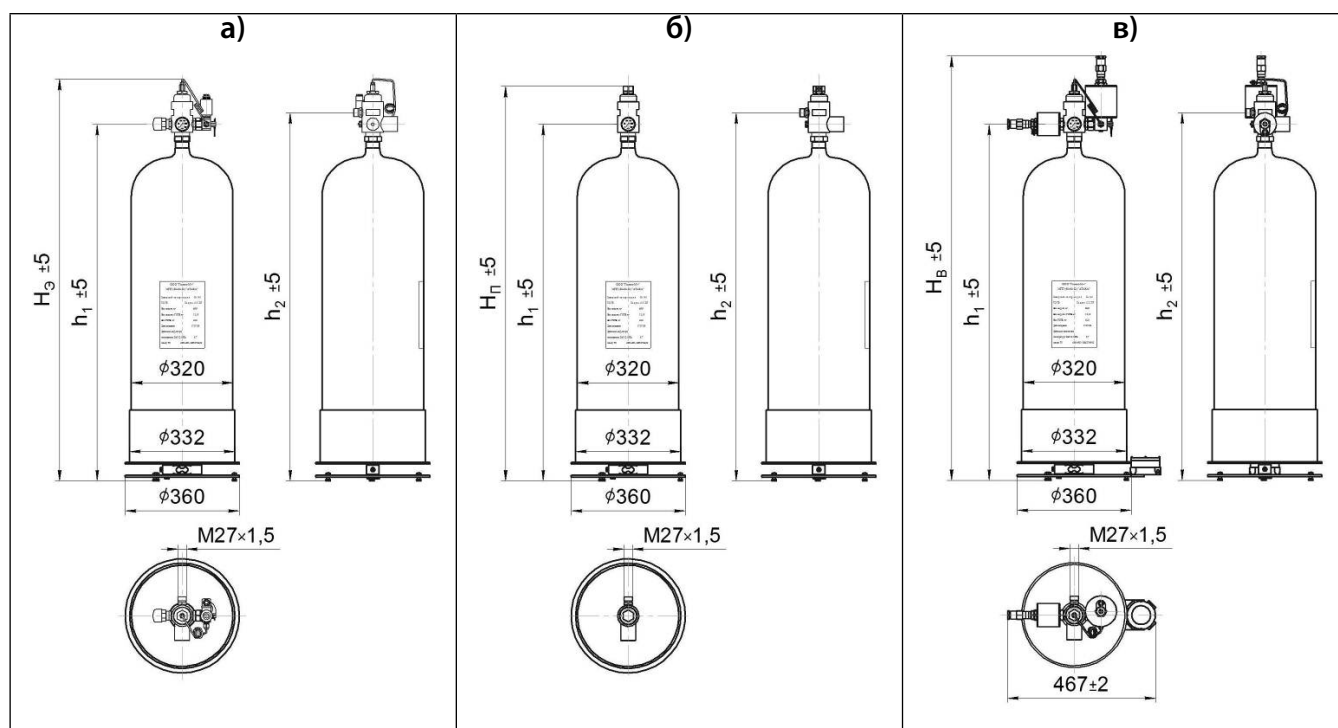
Рисунок 1.22 – МГП (150-60(80,100)-15), основанные на стальных цельнотянутых баллонах: а) с электрическим и ручным пуском; б) с пневмопуском; в) взрывозащищенный
