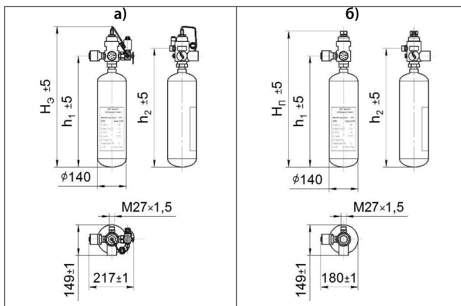
Рисунок 1.27 – МГП (150-5,10-15), основанные на стальных цельнотянутых баллонах: а) с электрическим и ручным пуском; б) с пневмопуском
