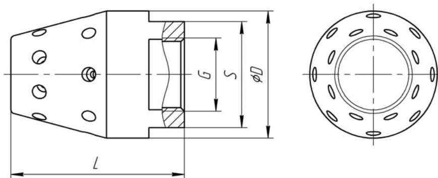
Рисунок 4.4 – Общий вид распылителя
