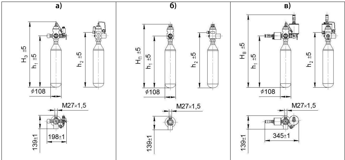
Рисунок 1.10 – МГП (150-2(3)-15), основанные на стальных цельнотянутых баллонах: а) с электрическим и ручным пуском; б) с пневмопуском; в) взрывозащищенный
