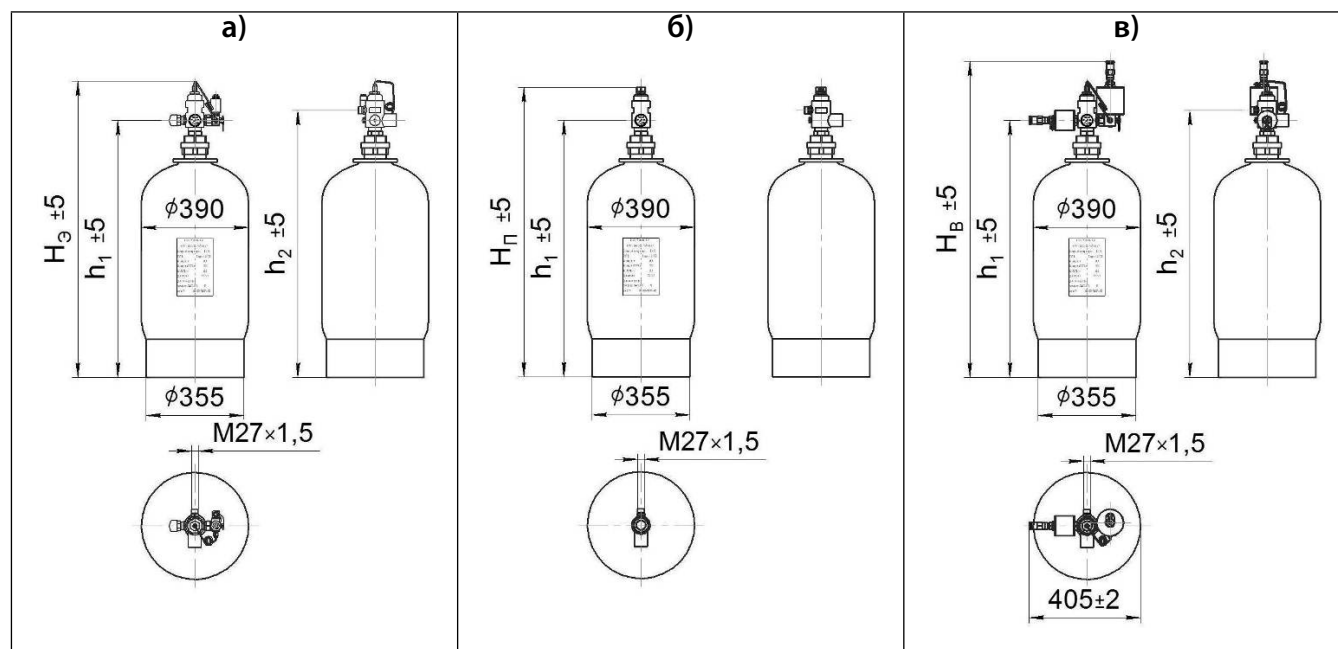
Рисунок 1.15 – МГПи (150-А-15), основанные на металлокомпозитных баллонах а) с электрическим и ручным пуском; б) с пневмопуском; в) взрывозащищенный
