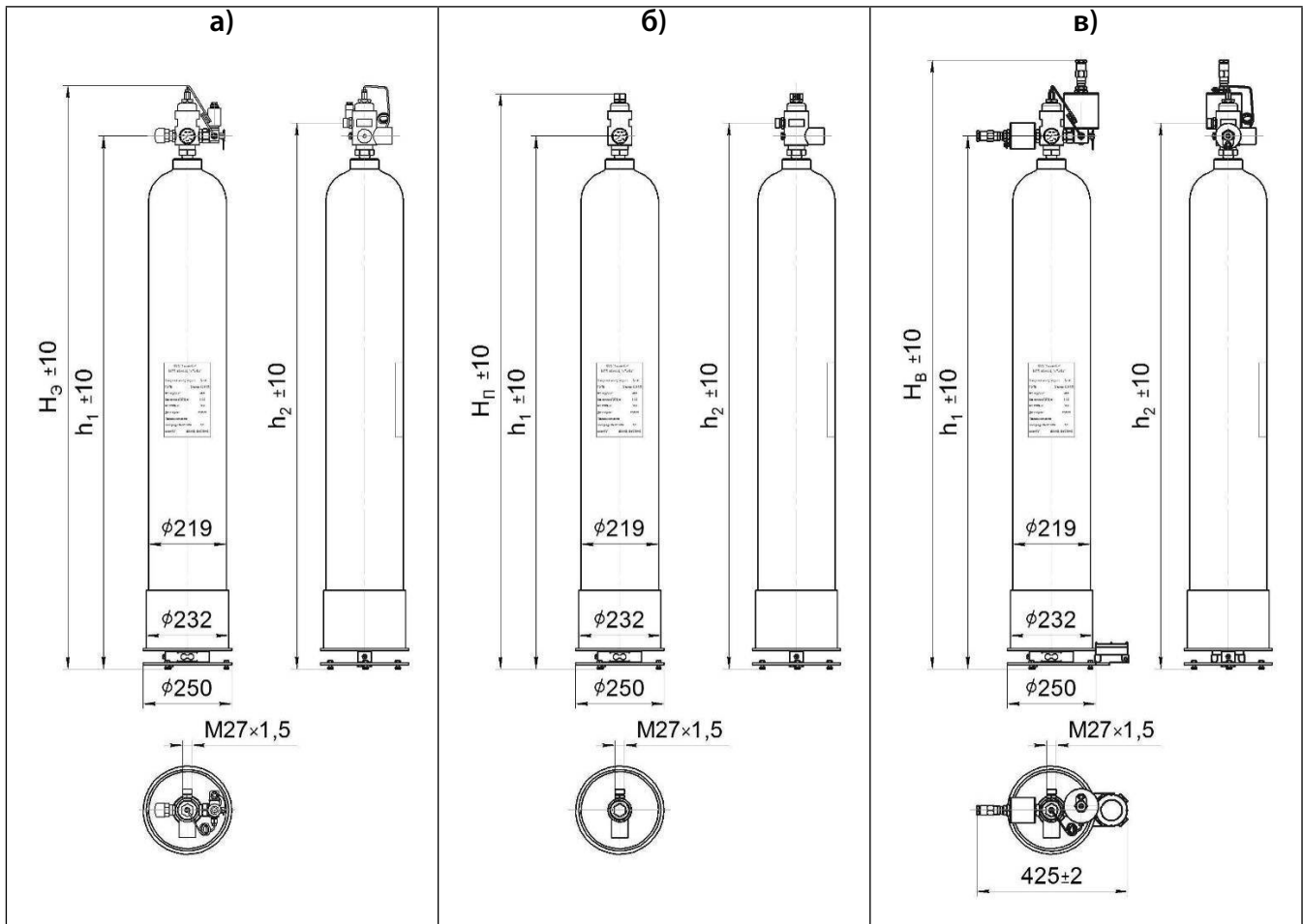
Рисунок 1.23 – МГП (150-40-15), основанные на стальных цельнотянутых баллонах: а) с электрическим и ручным пуском; б) с пневмопуском; в) взрывозащищенный
