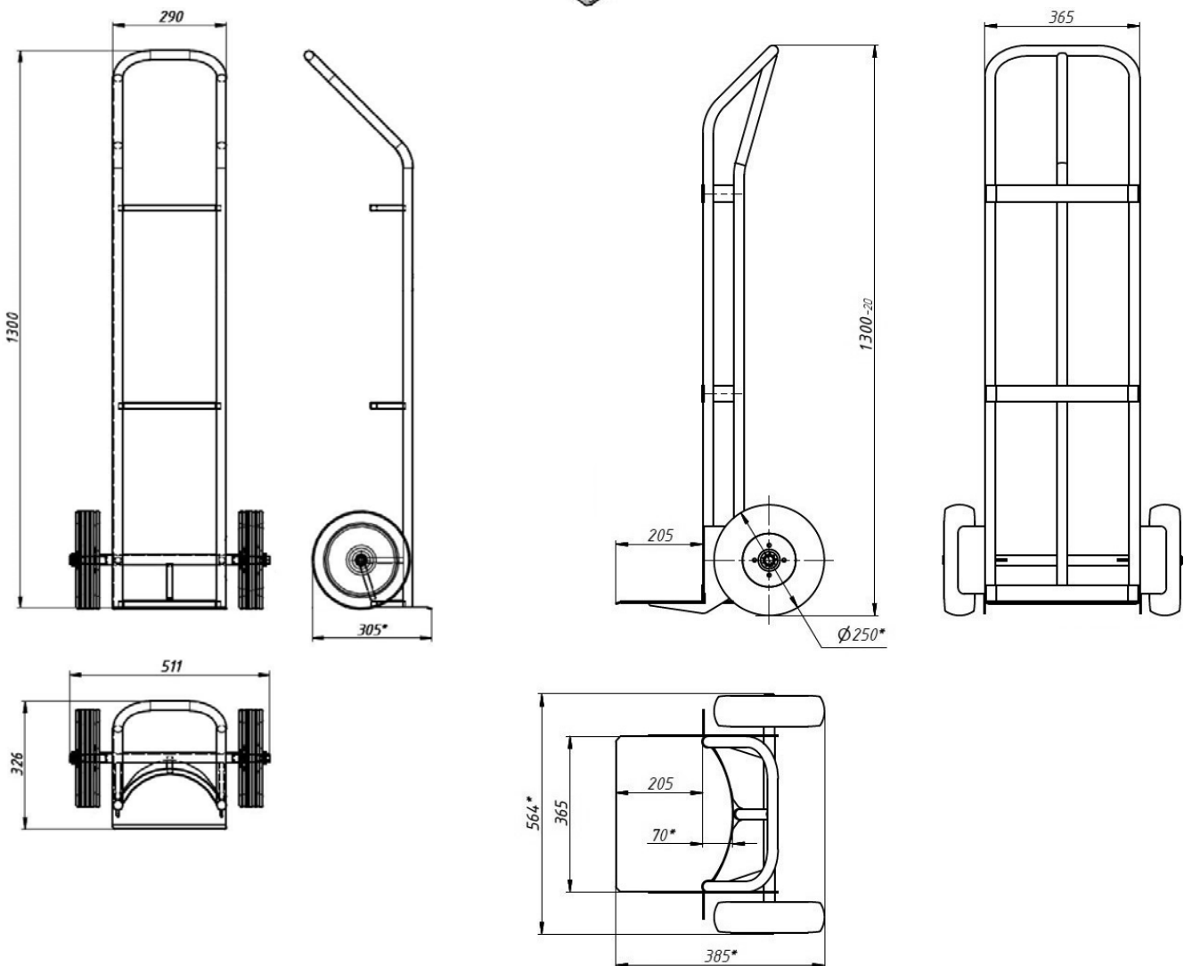
Рисунок 8.3 – Габаритные размеры тележки
