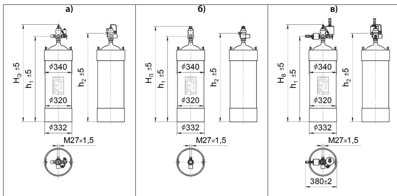
Рисунок 1.14 – МГПи (150-А-15), основанных на стальных цельнотянутых баллонах: а) с электрическим и ручным пуском; б) с пневмопуском; в) взрывозащищенный
