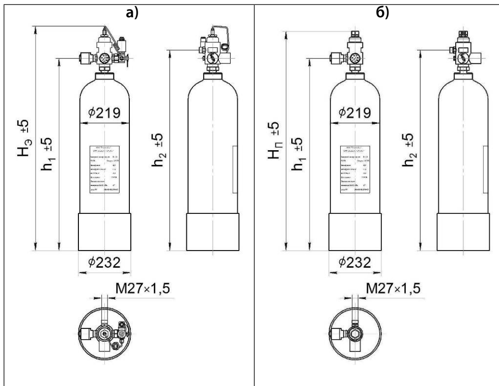
Рисунок 1.28 – МПП (150-20,25,40-15), основанные на стальных цельнотянутых баллонах: а) с электрическим и ручным пуском; б) с пневмопуском
