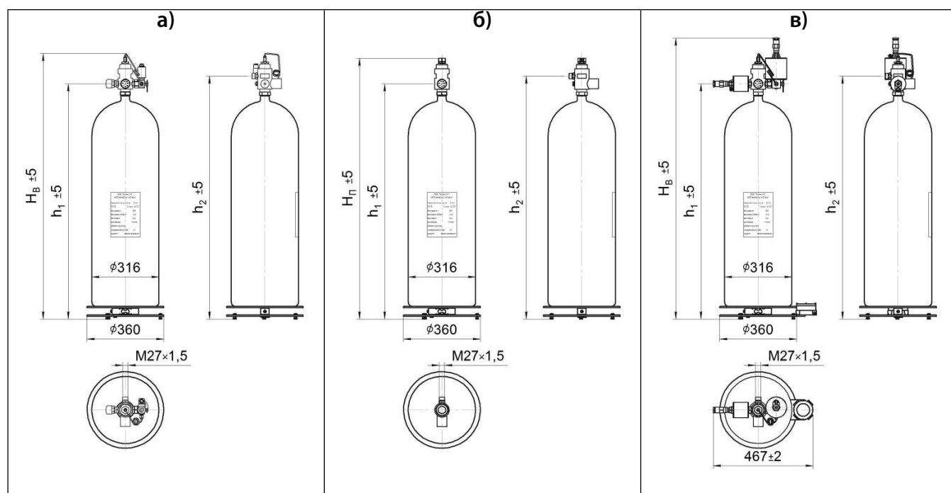
Рисунок 1.24 – МГП (150-А-15), основанные на стальных бесшовных баллонах: а) с электрическим и ручным пуском; б) с пневмопуском; в) взрывозащищенный
