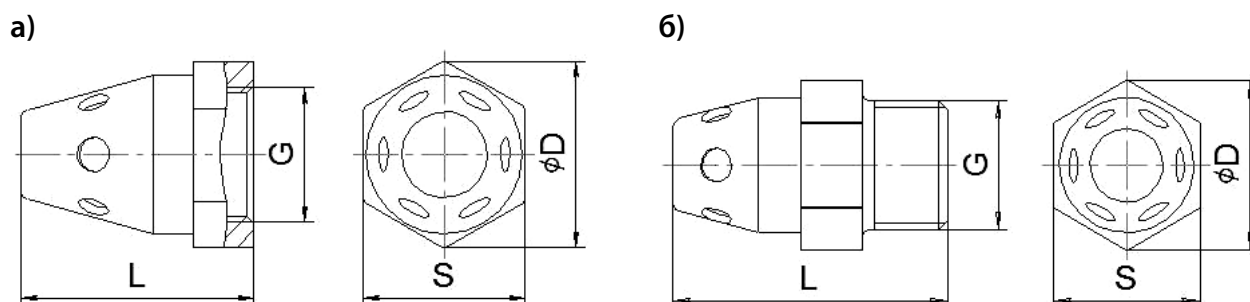
Рисунок 4.1 – Общий вид газовых распылителей:
