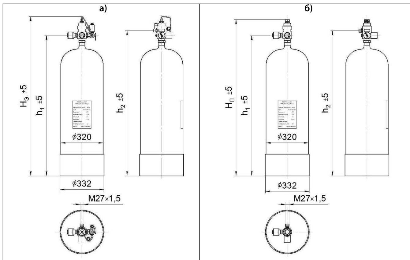
Рисунок 1.29 – МГП (150-А-15), основанные на стальных цельнотянутых баллонах: а) с электрическим и ручным пуском; б) с пневмопуском
