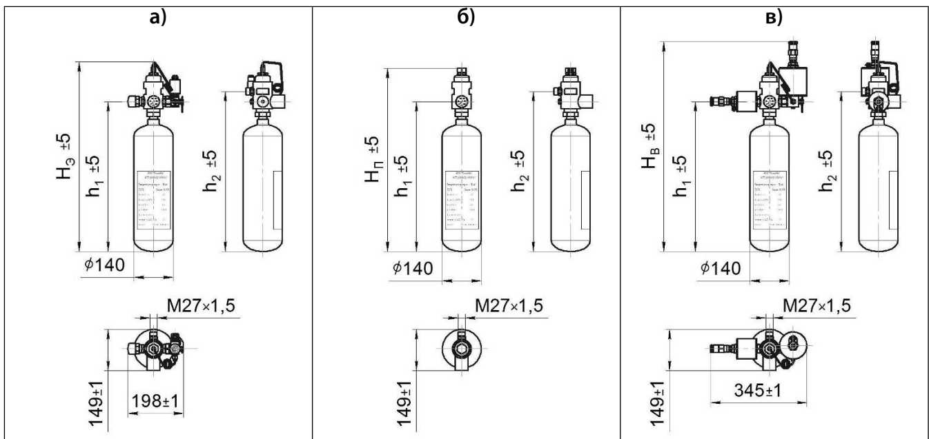
Рисунок 1.11 – МГП (150-5(10)-15), основанные на стальных цельнотянутых баллонах: а) с электрическим и ручным пуском; б) с пневмопуском; в) взрывозащищенный
