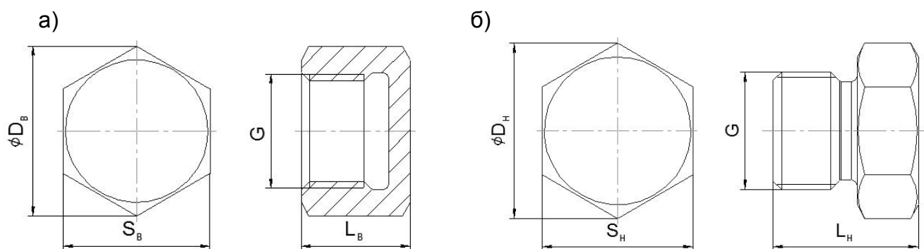
Рисунок 7.1 – Заглушка испытательная: а) с внутренней резьбой; б) с наружной резьбой
