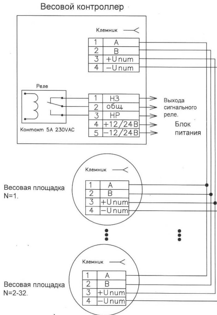
Рисунок 1.20 – Схема подключения УКМ-1 и УКМ-1в
